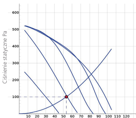
CIŚNIENIE/PRZEPIYW
