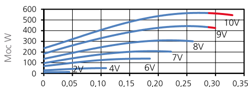
WYDAJNOŚĆ TEMPERATUROWA
