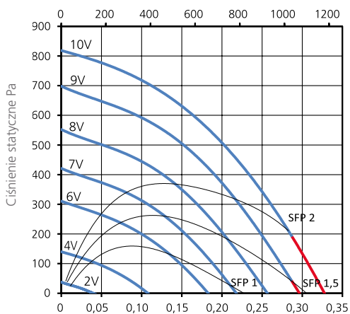
CIŚNIENIE/PRZEPŁYW
