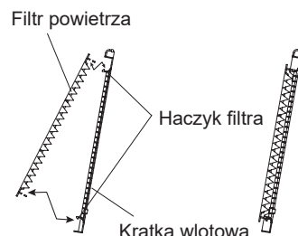
Kratka wlotowa
